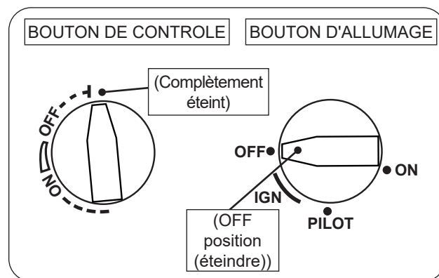
Fig. 51-2 Arrêt manuel
