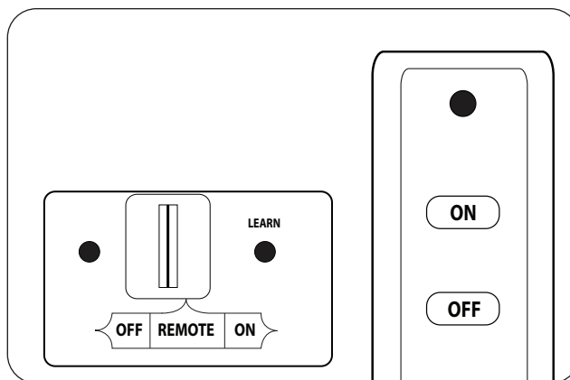
Fig. 46-2 Arrêt à distance
