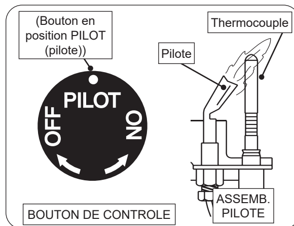
Fig. 53-1 Éclairage pilote
